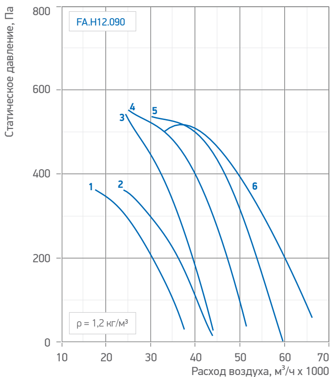
Табл. 30. Аэродинамические и акустические характеристики вентиляторов /FA.H12.090 (100_4)
