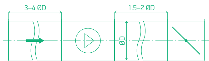
Схема 28. Монтаж в воздуховодах с элементами регулирования потока
