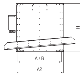
Схема 51. Станок монтажный с клапаном для скатной кровли TSA.V_, TSC.V_, TSE.V_
