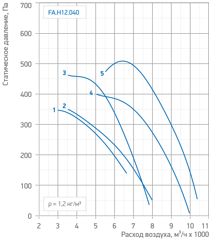
Табл. 25. Аэродинамические и акустические характеристики вентиляторов /FA.H12.040 (045)
