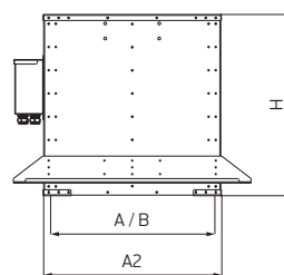
Схема 52. Станок монтажный с клапаном для плоской кровли TSA.V_, TSC.V_, TSE.V_
