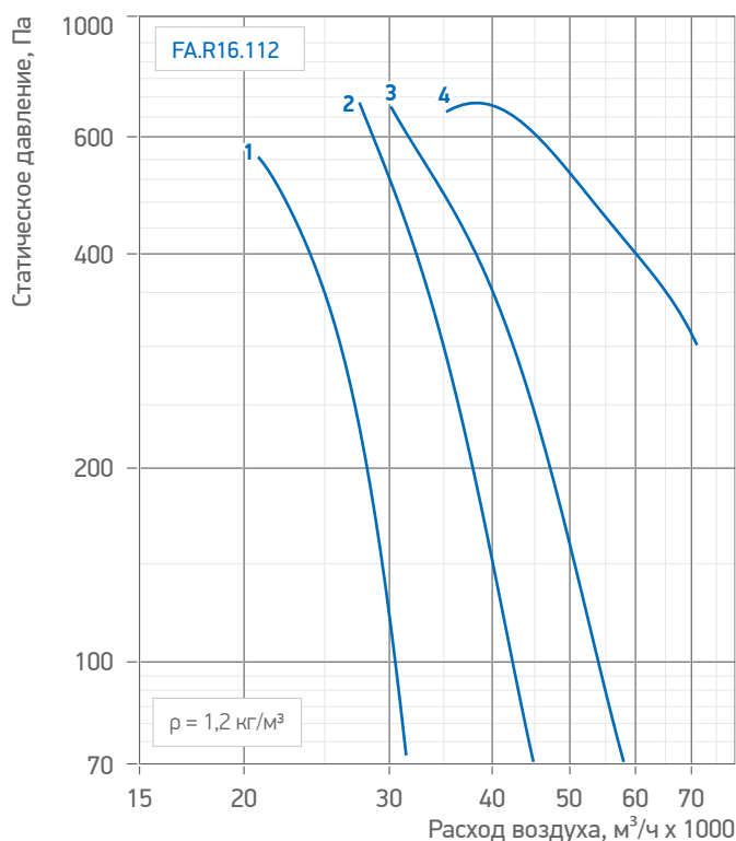
Гр. 17. Аэродинамические характеристики вентилятора /FA.R16.112
