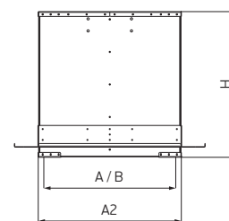
Схема 54. Станок монтажный с обратным клапаном вытяжка для плоской кровли TSA.B_, TSC.B_, TSE.B_
