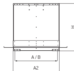
Схема 50. Стакан монтажный для плоской кровли TSA.N_, TSC.N_, TSE.N_
