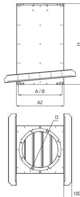
Схема 62. Станок монтажный с шумоглушителем и обратным клапаном для плоской кровли TSB.B_, TSD.B_, TSF.B_
