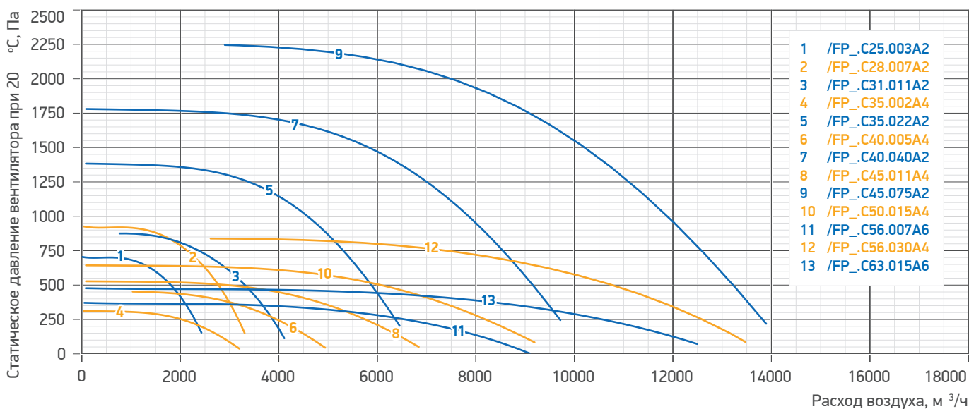
Гр. 2. Аэродинамические характеристики вентиляторов LM SAUGER /FP_ (продолжение)
