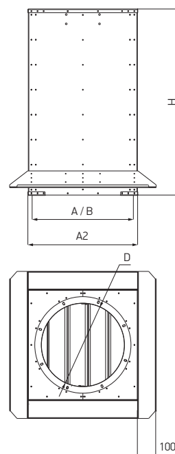
Схема 62. Станок монтажный с шумоглушителем и обратным клапаном для плоской кровли TSB.B_, TSD.B_, TSF.B_
