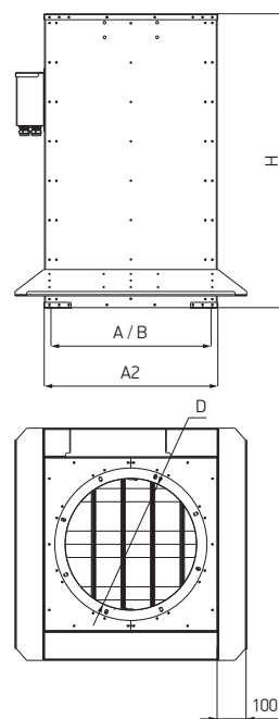
Схема 60. Станок монтажный с шумоглушителем и клапаном для плоской кровли TSB.V_, TSD.V_, TSF.V_
