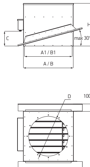
Схема 65. Иллюстрация исполнения стакана монтажного для скатной кровли TSA.F2, TSE.F2, TSC.F2
