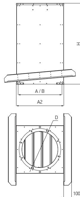
Схема 64. Станок монтажный с шумоглушителем и обратным клапаном для плоской кровли TSB.C_, TSD.C_, TSF.C_
