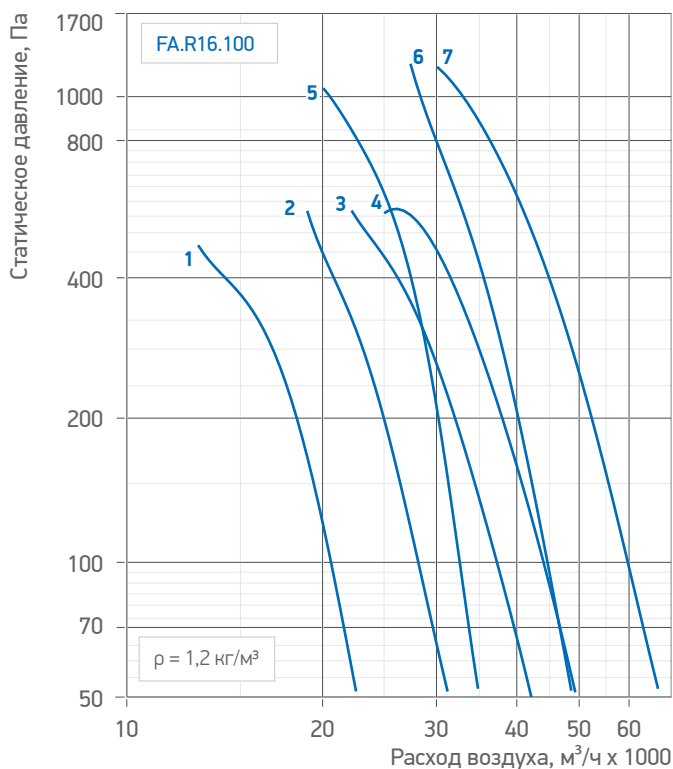
Гр. 16. Аэродинамические характеристики вентилятора /FA.R16.100
