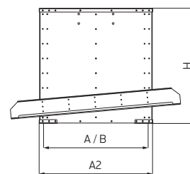
Схема 53. Станок монтажный с обратным клапаном вытяжка для скатной кровли TSA.B_, TSC.B_, TSE.B_
