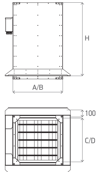
Схема 17. /TSSn.V4
