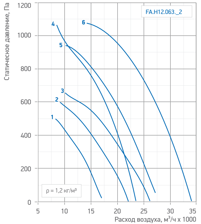
Гр. 24. Аэродинамические характеристики вентилятора /FA.H12.063_2
