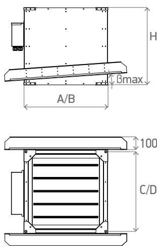
Табл. 5. Габаритные и присоединительные размеры монтажных стаканов /TSNn.B, /TSNn.N
