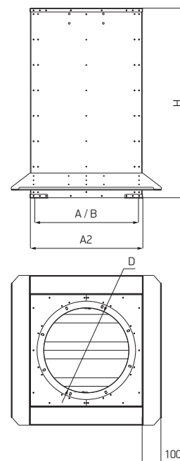
Схема 58. Станок монтажный с шумоглушителем для плоской кровли TSB.N_, TSD.N_, TSF.N_
