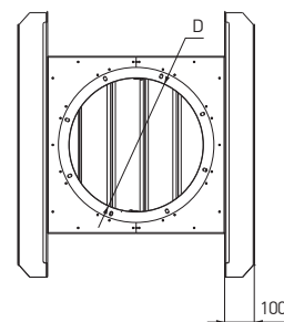
Схема 54. Станок монтажный с обратным клапаном вытяжка для плоской кровли TSA.B_, TSC.B_, TSE.B_
