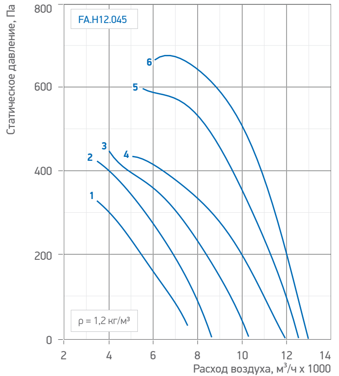
Табл. 25. Аэродинамические и акустические характеристики вентиляторов /FA.H12.040 (045)
