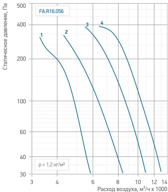
Гр. 11. Аэродинамические характеристики вентилятора /FA.R16.056
