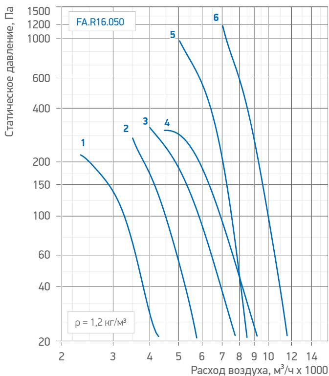
Гр. 10. Аэродинамические характеристики вентилятора /FA.R16.050
