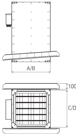
Табл. 7. Габаритные и присоединительные размеры монтажных стаканов /TSS_
