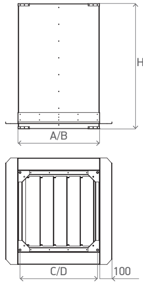
Схема 16. /TSSn.V2
