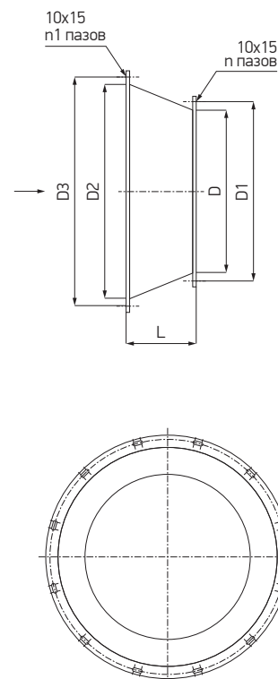
Схема 40. Конфузор на всасе
