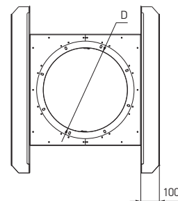
Схема 50. Стакан монтажный для плоской кровли TSA.N_, TSC.N_, TSE.N_
