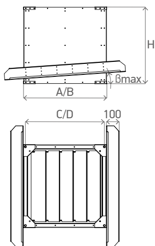
Схема 9. /TSNn.N2
