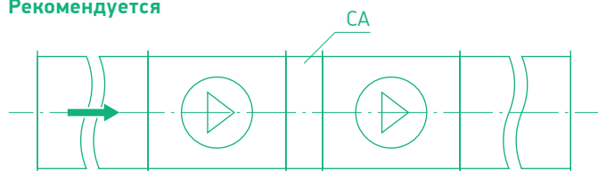
Схема 35. Последовательная установка вентиляторов
