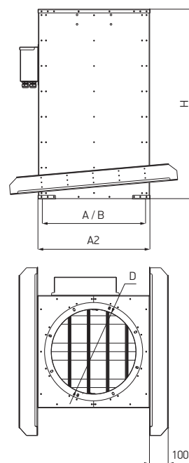
Схема 60. Станок монтажный с шумоглушителем и клапаном для плоской кровли TSB.V_, TSD.V_, TSF.V_
