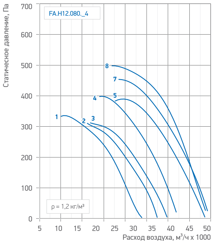
Табл. 29. Аэродинамические и акустические характеристики вентилятора /FA.H12.080
