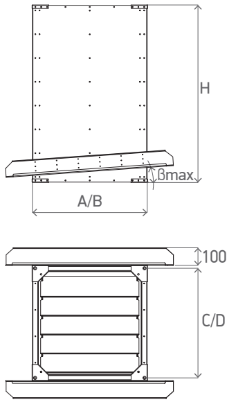
Схема 15. /TSSn.N4
