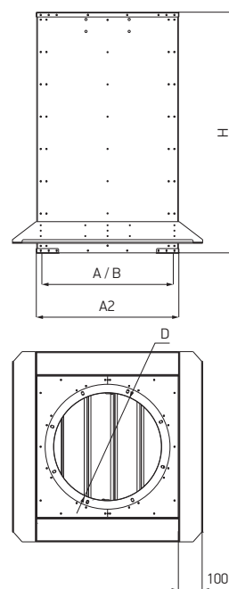
Схема 64. Станок монтажный с шумоглушителем и обратным клапаном для плоской кровли TSB.C_, TSD.C_, TSF.C_
