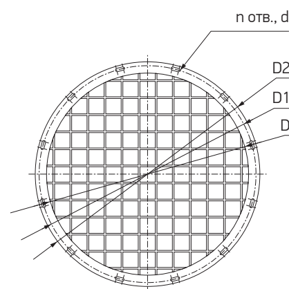
Схема 47. Защитная сетка
