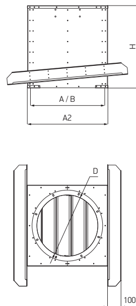
Схема 56. Станок монтажный с обратным клапаном приток для плоской кровли TSA.C_, TSC.C_, TSE.C_
