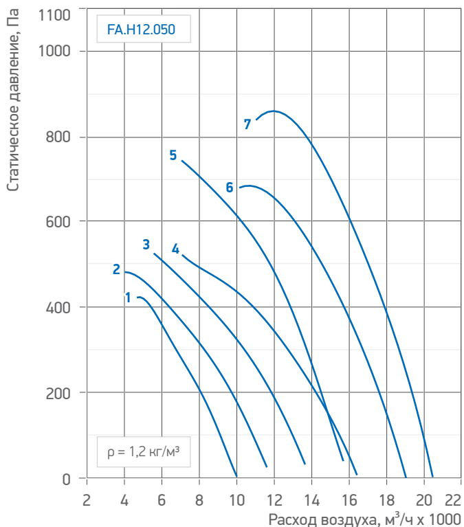
Табл. 26. Аэродинамические и акустические характеристики вентиляторов /FA.H12.050 (056)
