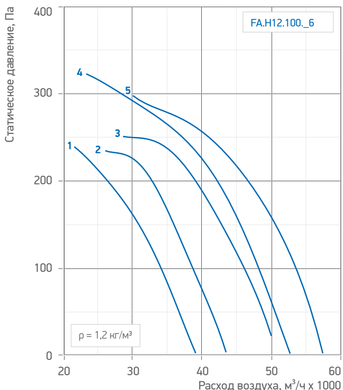
Табл. 31. Аэродинамические и акустические характеристики вентиляторов /FA.H12.100_6 (112_4)
