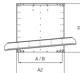
Схема 49. Стакан монтажный для скатной кровли TSA.N_, TSC.N_, TSE.N_
