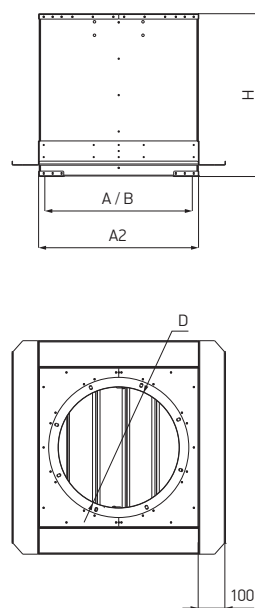
Схема 56. Станок монтажный с обратным клапаном приток для плоской кровли TSA.C_, TSC.C_, TSE.C_
