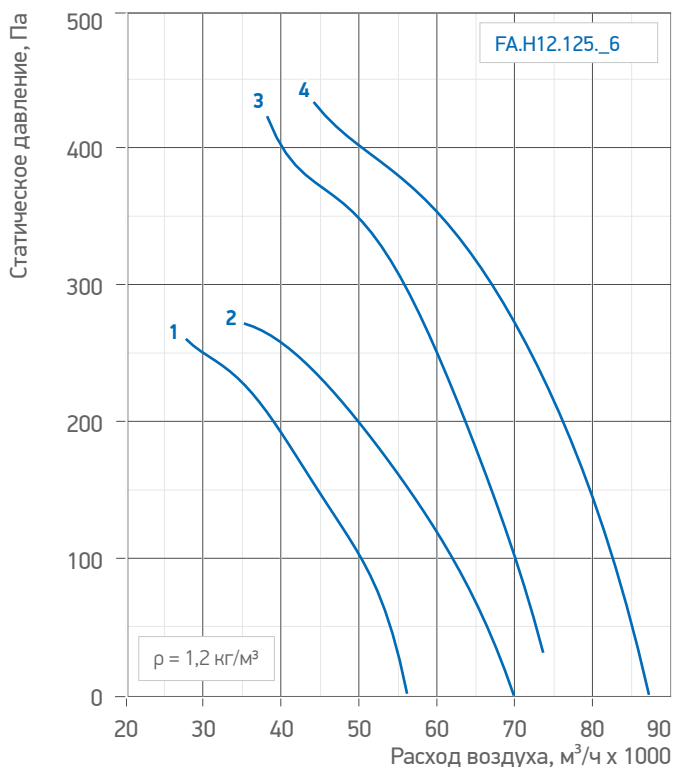
Табл. 33. Аэродинамические и акустические характеристики вентилятора /FA.H12.125_6
