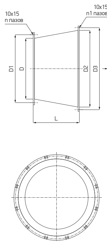
Схема 41. Диффузор на выхлопе
