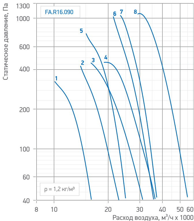
Табл. 21. Аэродинамические и акустические характеристики вентиляторов /FA.R16.080 (090)
