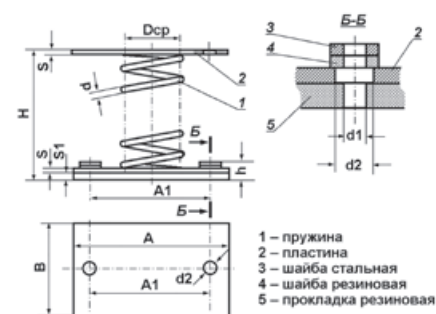
Схема 46. Виброизолятор
