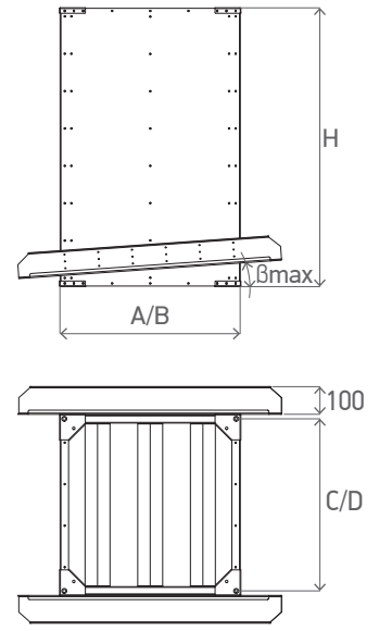
Схема 17. /TSSn.V4
