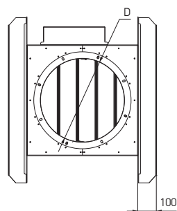
Схема 52. Станок монтажный с клапаном для плоской кровли TSA.V_, TSC.V_, TSE.V_
