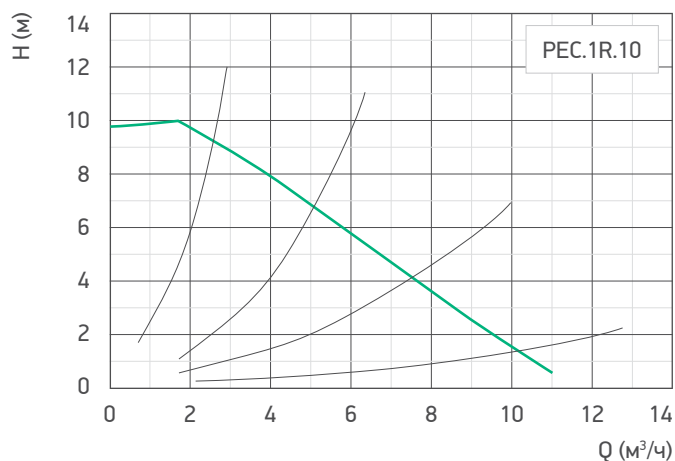
Гр. 14. Гидравлические характеристики насоса /PEC.1R.10
