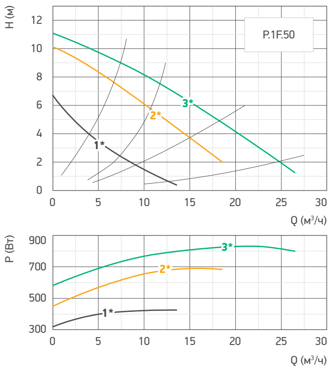
Гр. 7. Гидравлические характеристики насоса /P.1F.50
