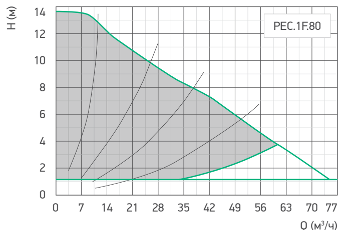
Гр. 17. Гидравлические характеристики насоса /PEC.1F.80
