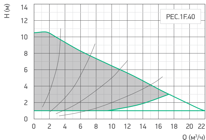
Гр. 15. Гидравлические характеристики насоса /PEC.1F.40
