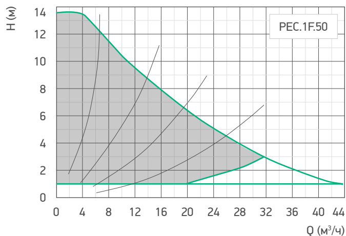
Гр. 16. Гидравлические характеристики насоса /PEC.1F.50
