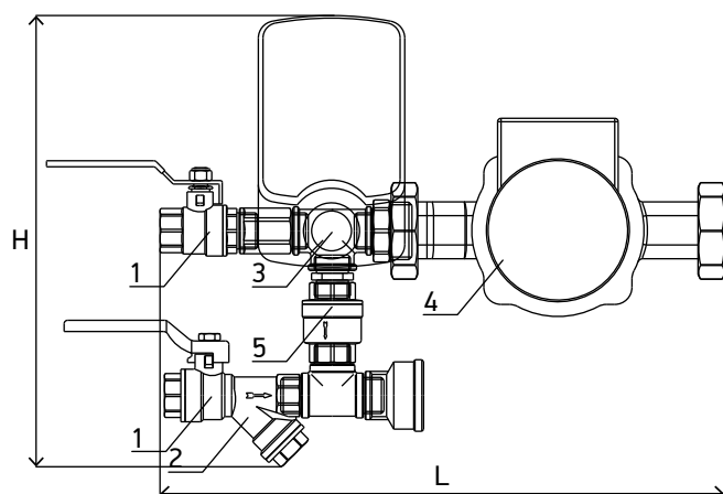
Схема 4. Смесительный узел /MUB
