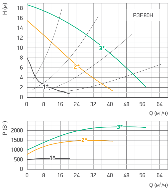
Гр. 11. Гидравлические характеристики насоса /P.3F.80H
