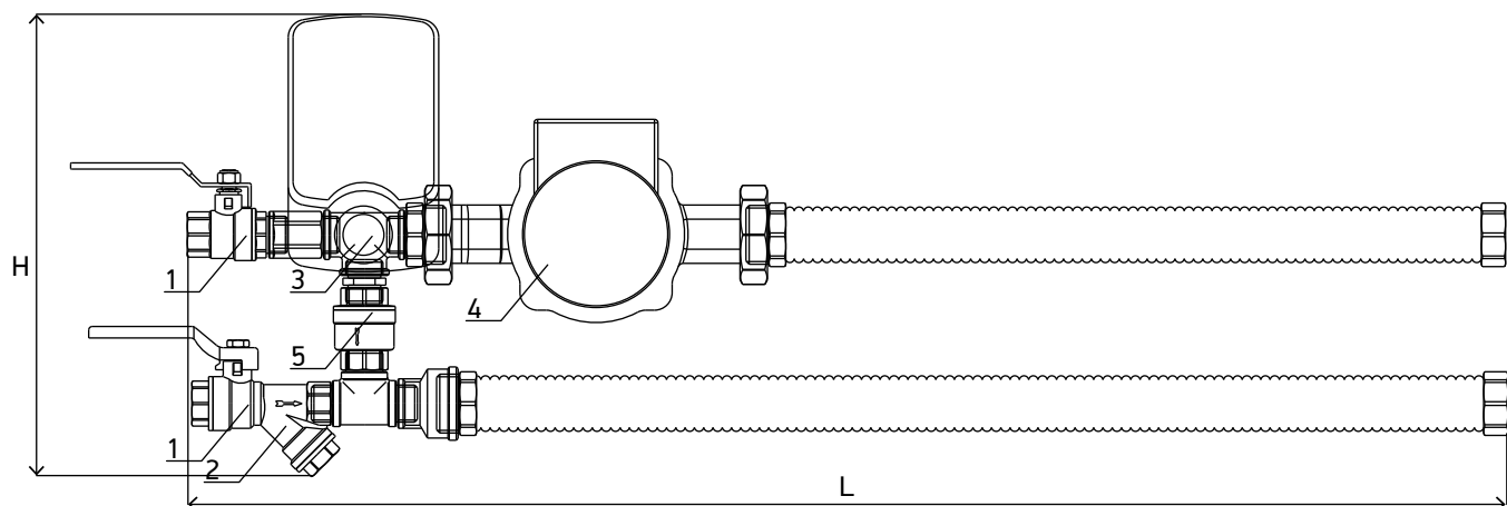
Схема 6. Смесительный узел /MUB...CP
