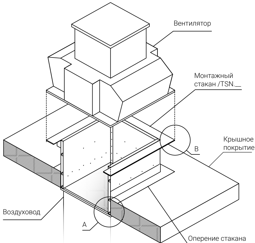
Схема 5. Узел крепления монтажного стакана к воздуховоду, вентилятора к монтажному стакану
