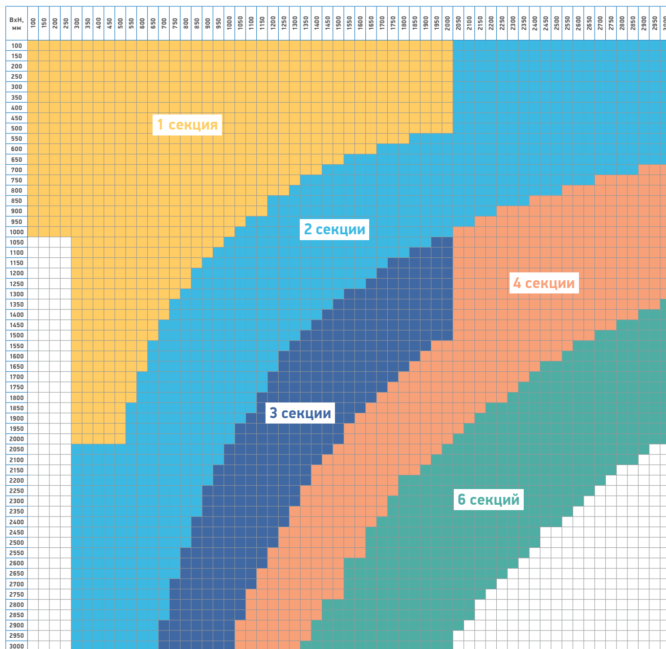
Табл. 52. Секционность решеток в канальном исполнении в зависимости от параметров сечения клапана
