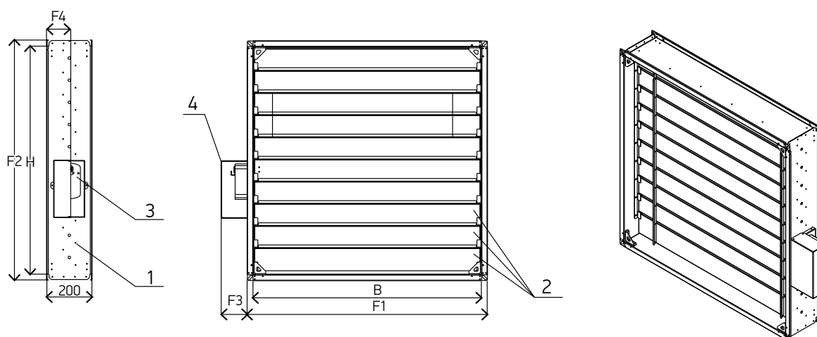
Схема 24. Противопожарные каналные клапаны прямоугольного сечения многолопаточные EI60, EI90
