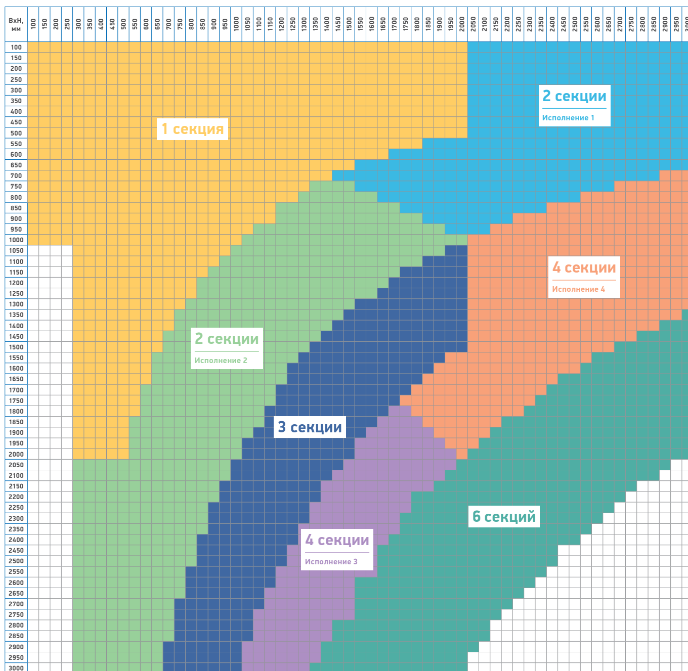
Табл. 16. Исполнения клапана (количество секций) в зависимости от параметров сечения
