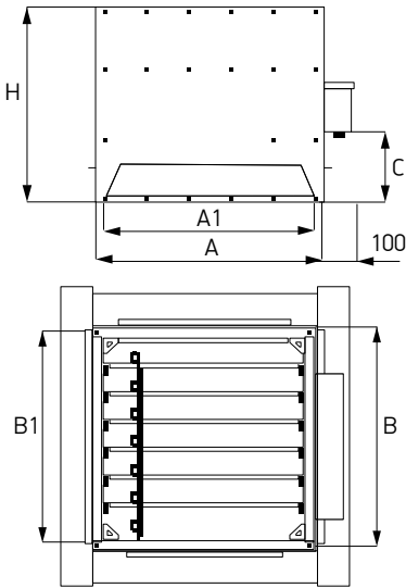
Схема 8. Поддон для сбора конденсата /APn.1
